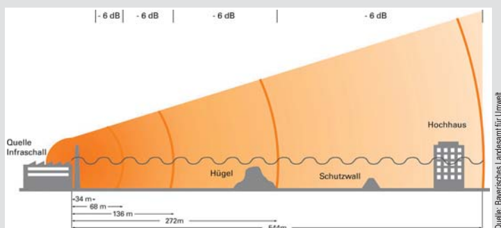
Dargestellt ist Infraschall von 10 Hertz mit einer Wellenlänge von 34 Metern
